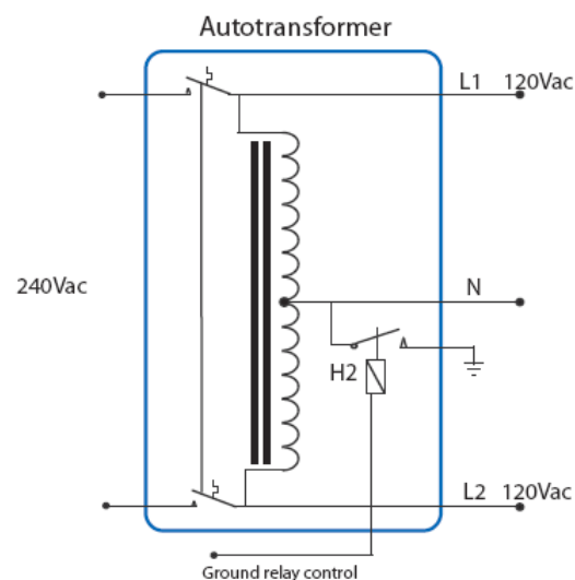
Autotransformador: diagrama esquemático
