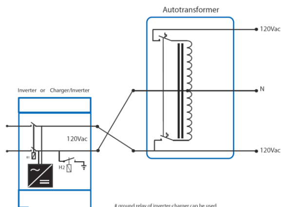
Autotransformador: diagrama esquemático
