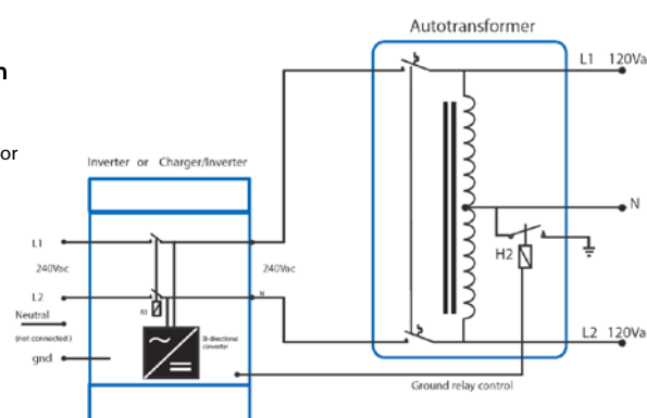
Figura 1: Alimentación de energía con fases separadas para cargas desequilibradas
